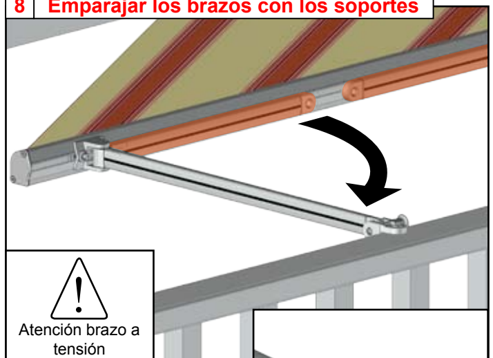
8 Emparajar los brazos con los soportes
