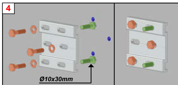
Fijación de los tornillos de Ø10mm. Kit de tornillos y tacos no incluidos.
