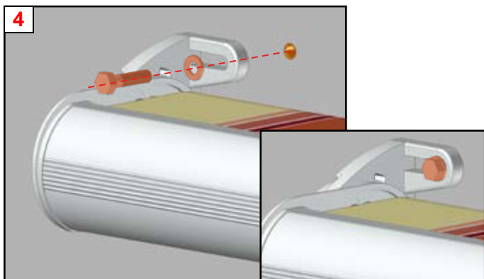
Fijación de los tornillos de Ø10mm. Kit de tornillos y tacos no incluidos.
